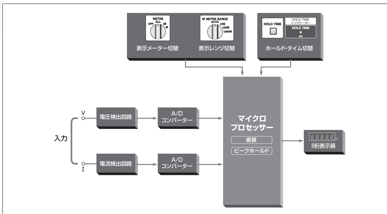
第2図 デジタル・パワーメーターのブロック・ダイアグラム
