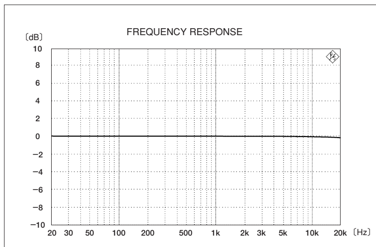
周波数特性
