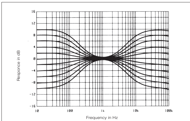
トーン・コントロール特性
