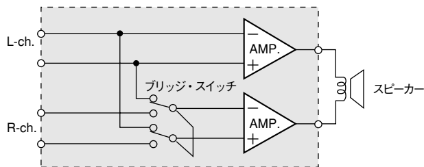
P-450のブリッジ接続回路 (バランス入力時、スイッチの位置はブリッジ接続側)
