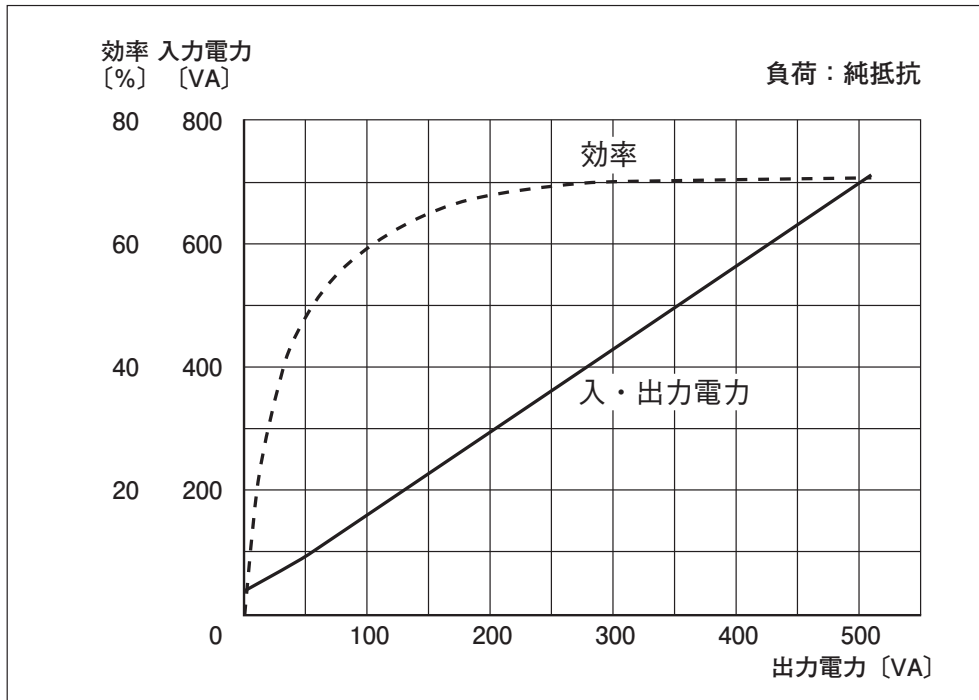
出力電力／効率・入力電力特性図
