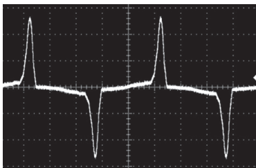
写真⑦ 電源ラインの電圧波形(ひずみ率: 約3%)
