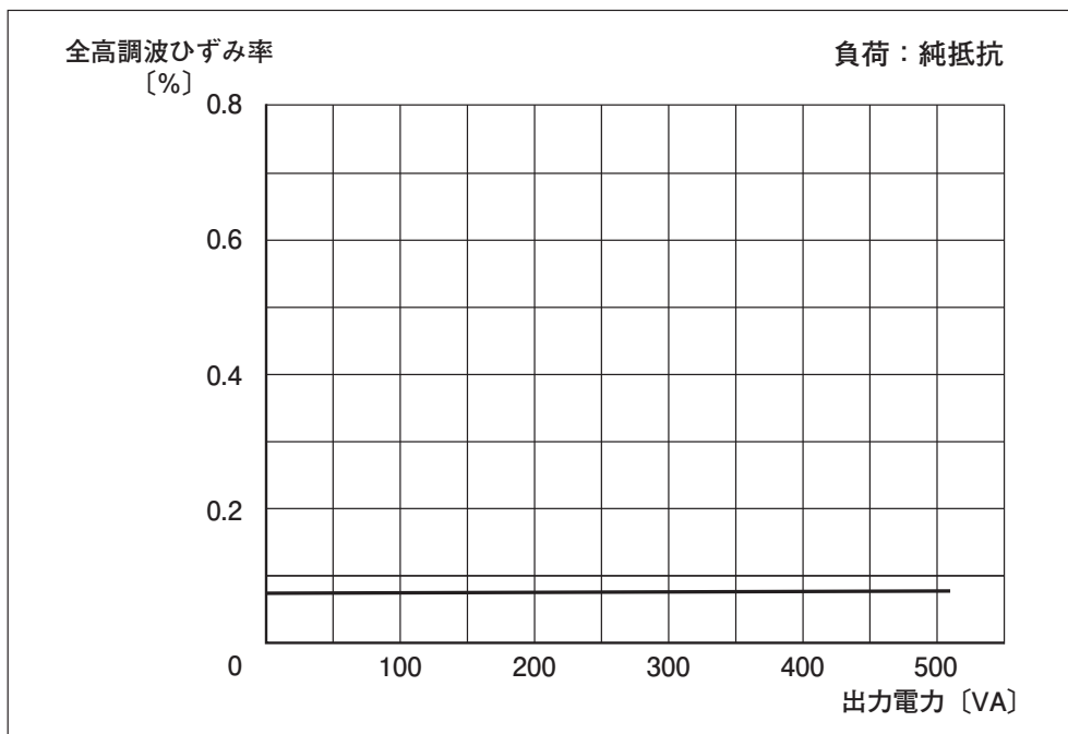
出力電力／全高調波ひずみ率特性図
