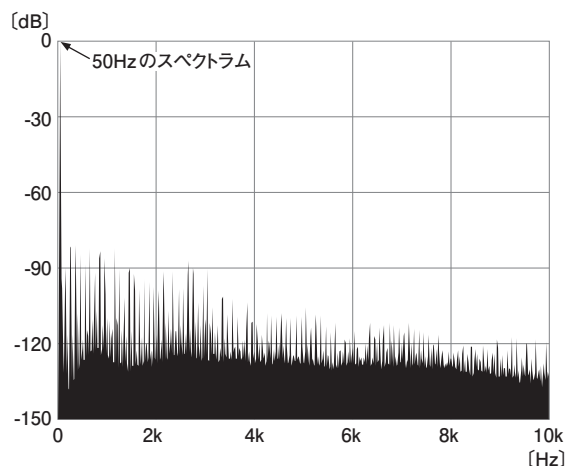
図2 PS-550出力(写真③)の周波数スペクトラム
