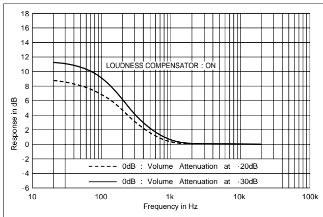
コンペ-ンセ-ター特性
