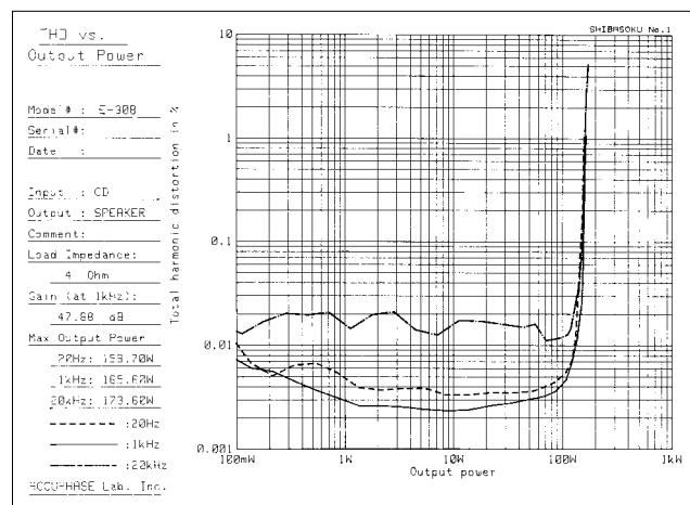
出力電力 / 全高調波ひずみ率特性 (4 負荷時)
