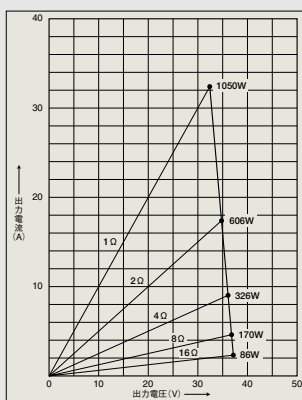
第2図 負荷インピーダンスに対する出力電力特性 (出力電圧/出力電流) *1Ωは音楽信号に限る
