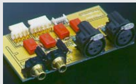
アンバランス入力端子と バランス入力コネクタ
