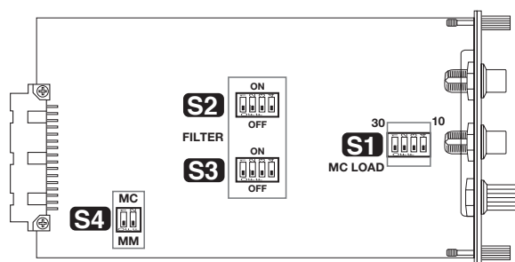
AD-20 部品面 (S1~S4のスイッチ位置を示す。)
